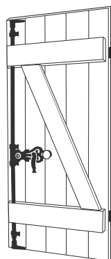
Panneau avec barres et écharpes.
