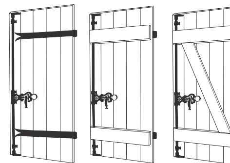
Panneau seul. Panneau avec barres. Panneau avec barres et écharpes.
